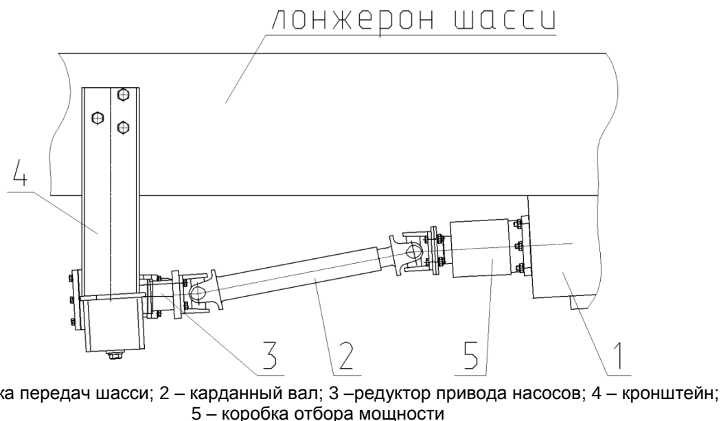
Рисунок 10 Установка привода насосов для шасси МАЗ 6303А3
