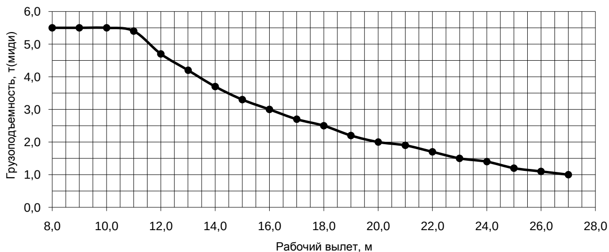
Грузовая характеристика L_{ст}=9,9 м. \kappa=10...12 . Опорный контур 4,1х2,3м., противовес G=1,7 т.
