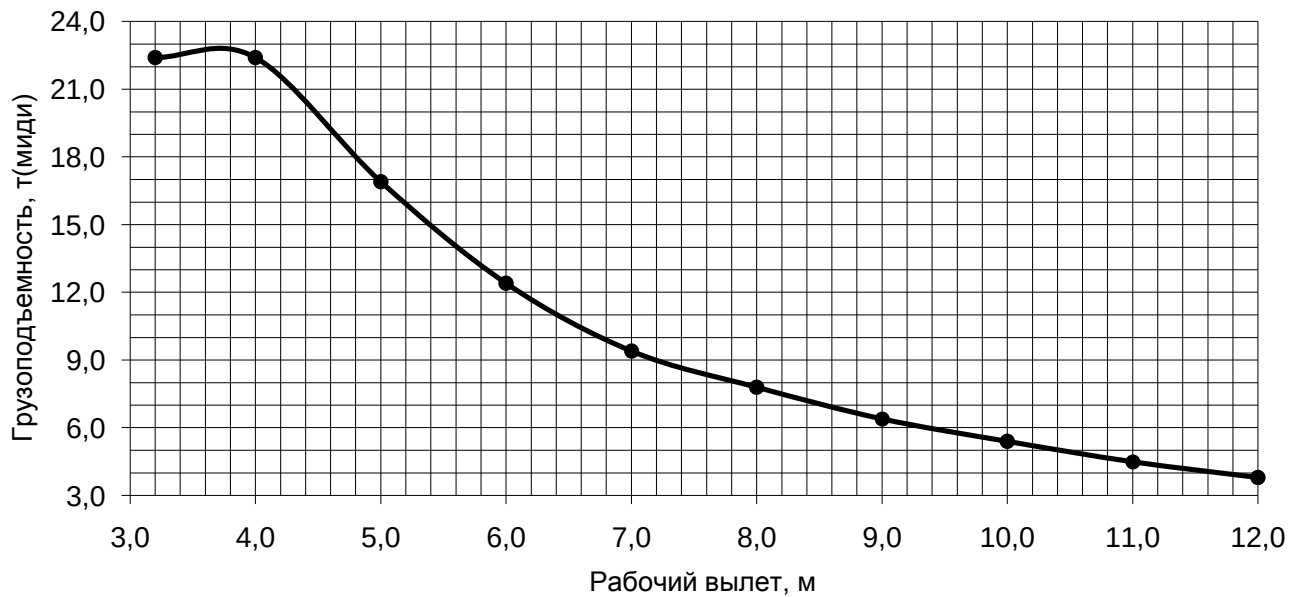
Грузовая характеристика L_{ст}=12,0-14,0 м. \kappa=10 , противовес G=1,7 т.
