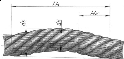
Волнистость каната
