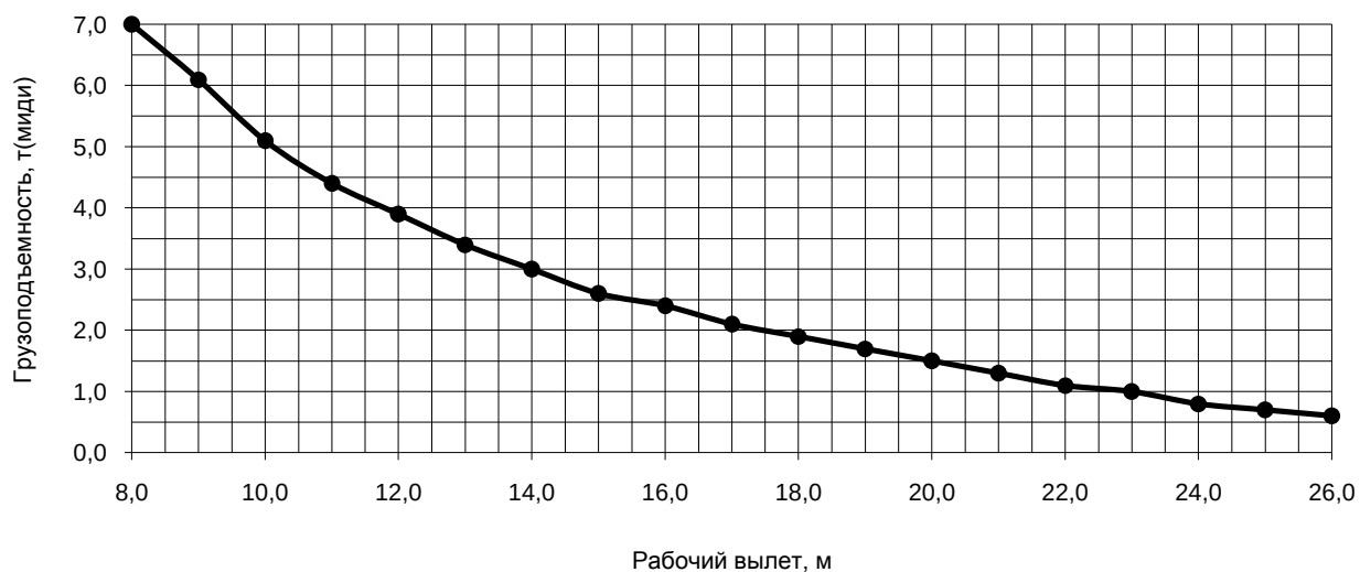
Грузовая характеристика. L_{ст}=26,0-28,0 м. \kappa=4 , противовес G=1,7 т.
