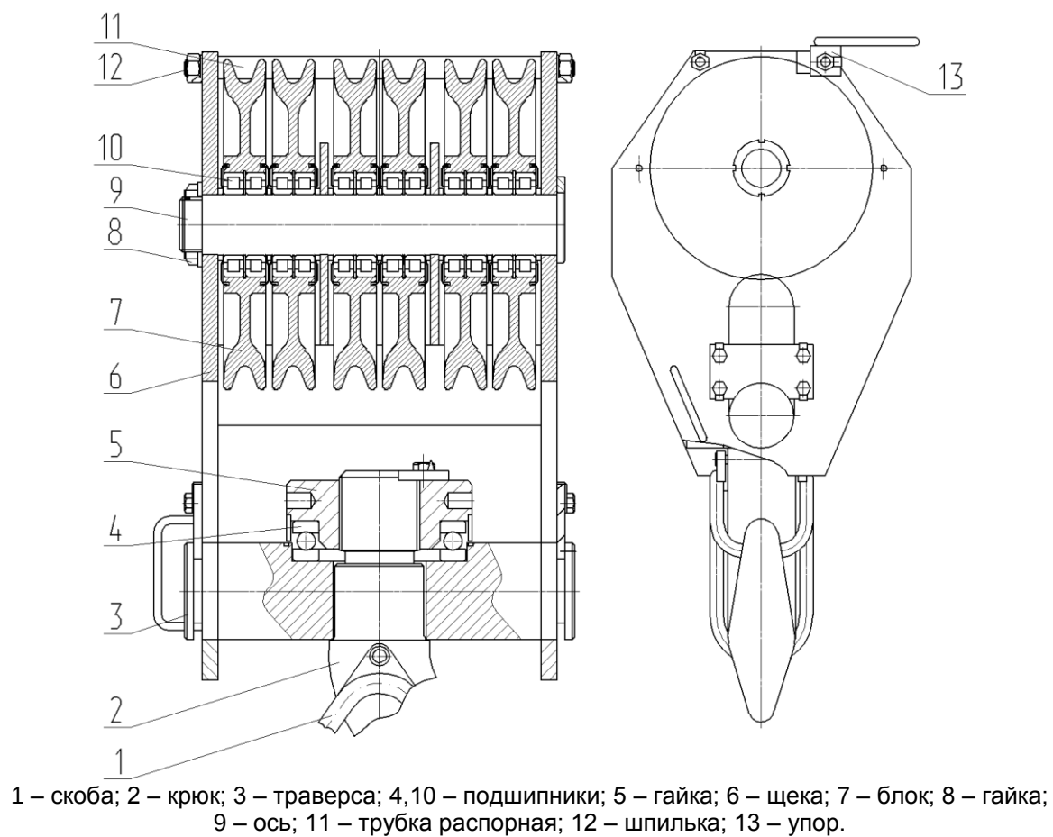
Рисунок 24 Обойма крюковая
