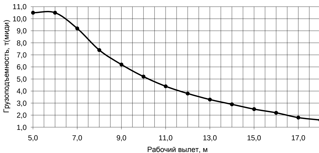
Грузовая характеристика Лст=18,0-20,0м. \kappa=4 , противовес G=1,7 т.
