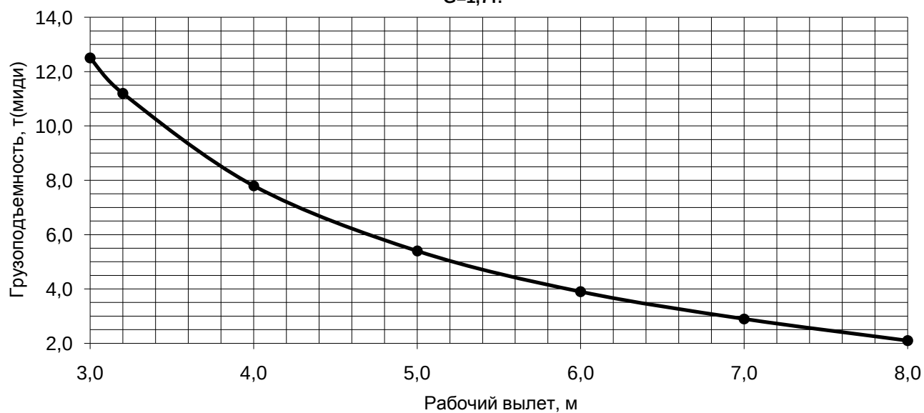
Грузовая характеристика L_{ст}=9,9 м. \kappa=10...12 . Опорный контур 4,1х2,3м., противовес G=1,7 т.
