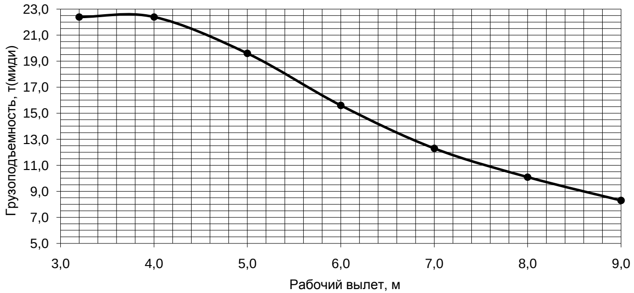
Грузовая характеристика. Лст=11,0-12,0м. \kappa=10 противовес G=4,2 т.
