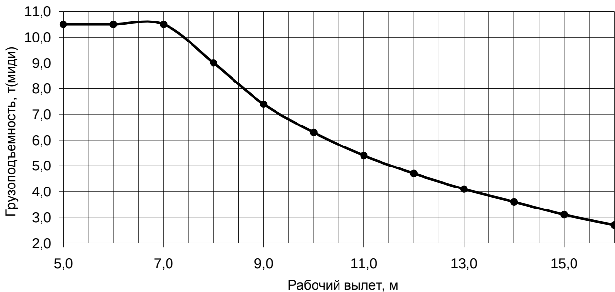
Грузовая характеристика. Лст=16,7-18,0м. \kappa=4 , противовес G=4,2 т.
