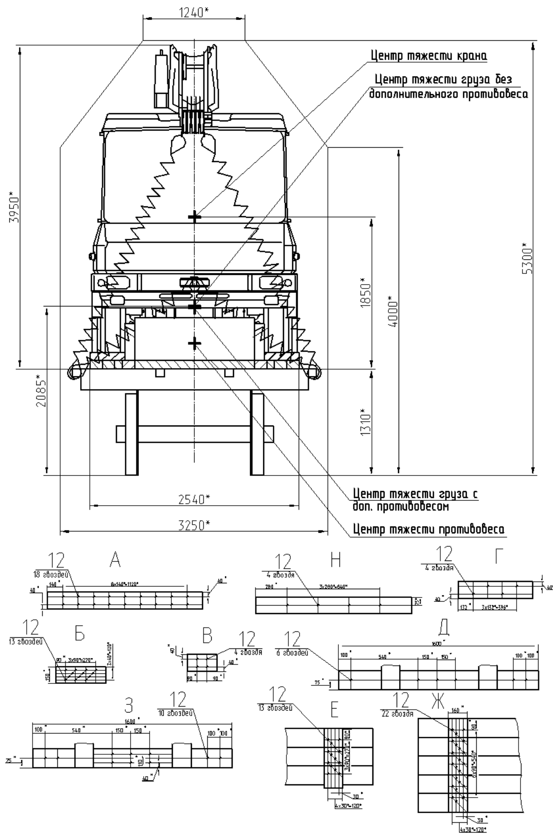
Рисунок 66 Схема отгрузки крана
