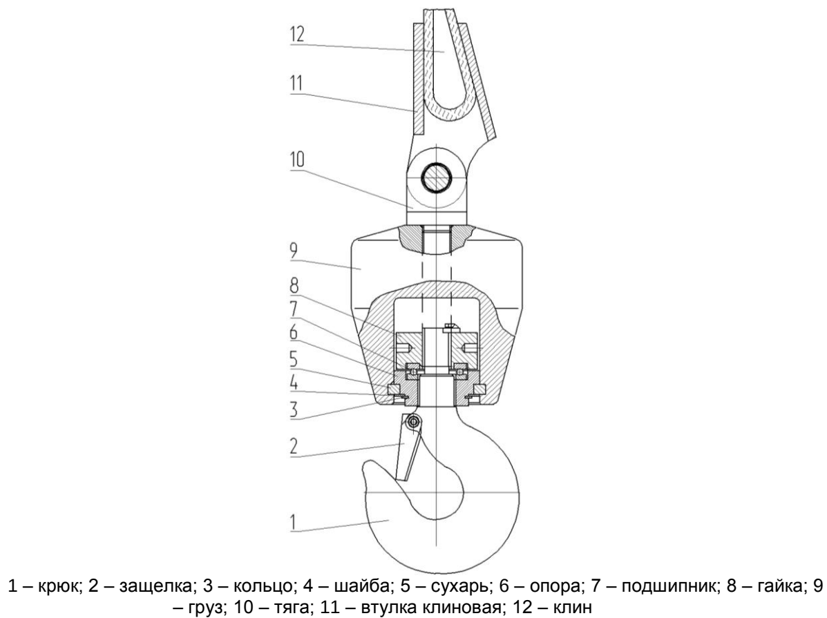
Рисунок 25 Обойма крюковая малая
