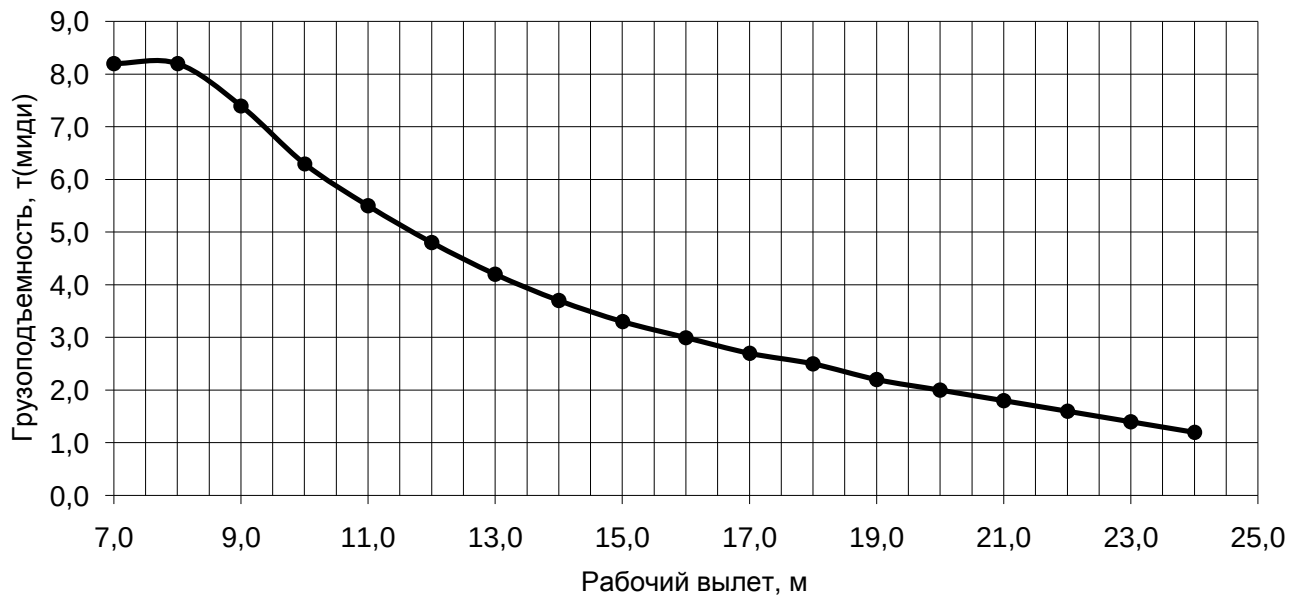
Грузовая характеристика. Лст=24,0-26,0м. \kappa=4 , противовес G=4,2 т.
