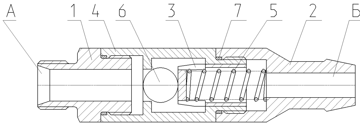
Рисунок 54 Клапан обратный
