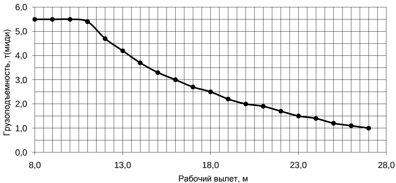
Грузовая характеристика Lст=9,9м. κ=10...12.Опорный контур 4,1х2,3м.,противовес G=4,2т.
