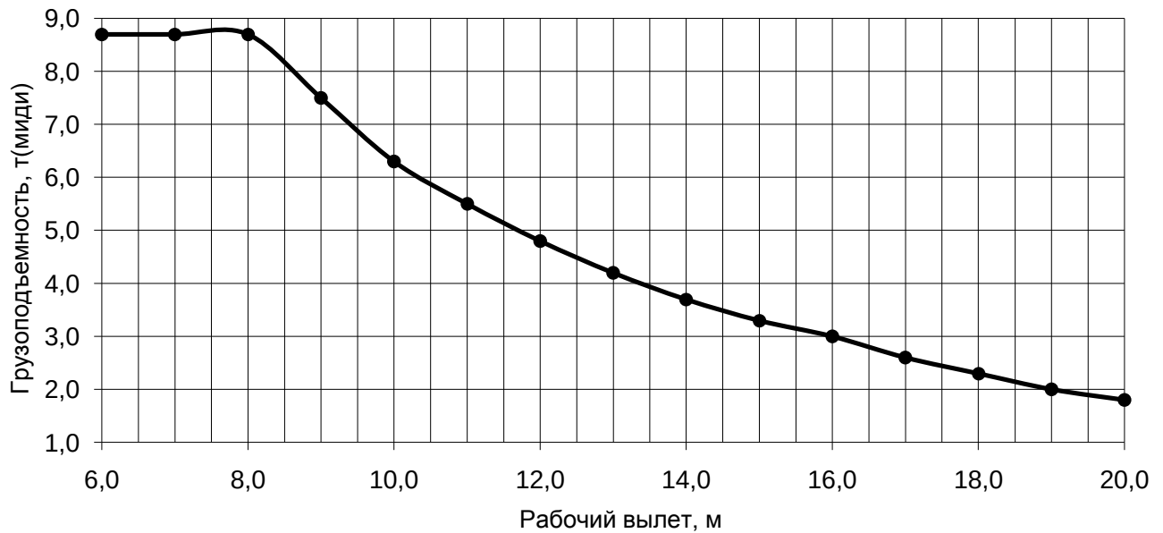
Грузовая характеристика. Лст=20,0-22,0м. \kappa=4 , противовес G=4,2 т.
