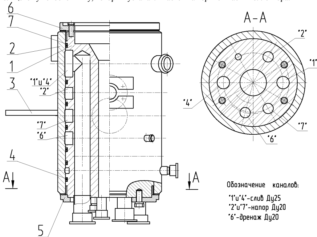
Рисунок 49 Центральный коллектор
