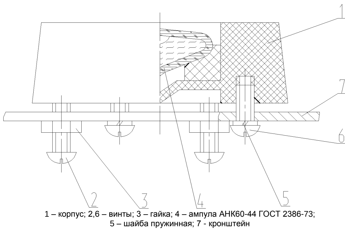
Рисунок 34 Креномер
