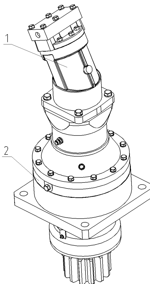
Рисунок 18 Механизм поворота
