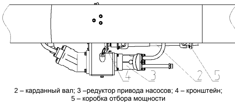
Рисунок 11 Установка привода насосов для шасси МАЗ 630333
