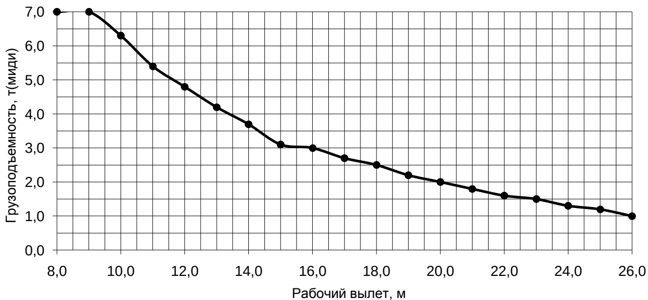
Грузовая характеристика. Lст=26,0-28,0м. κ=4, противовес G=4,2 т.
