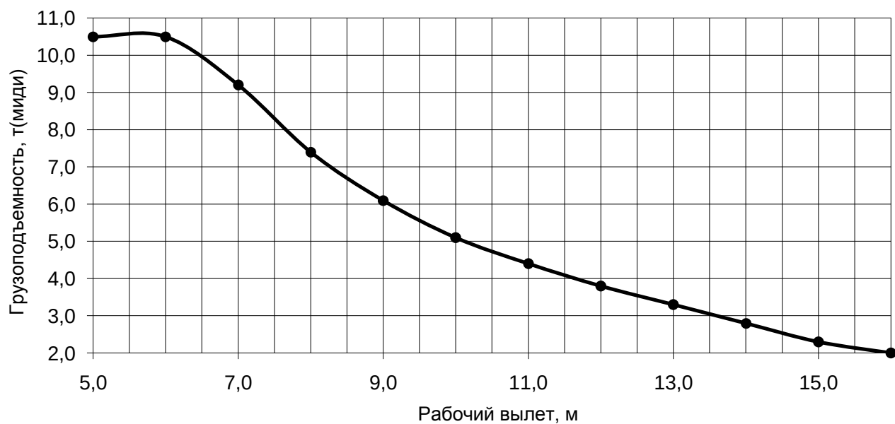
Грузовая характеристика Лст=16,7-18,0м. \kappa=4 , противовес G=1,7 т.
