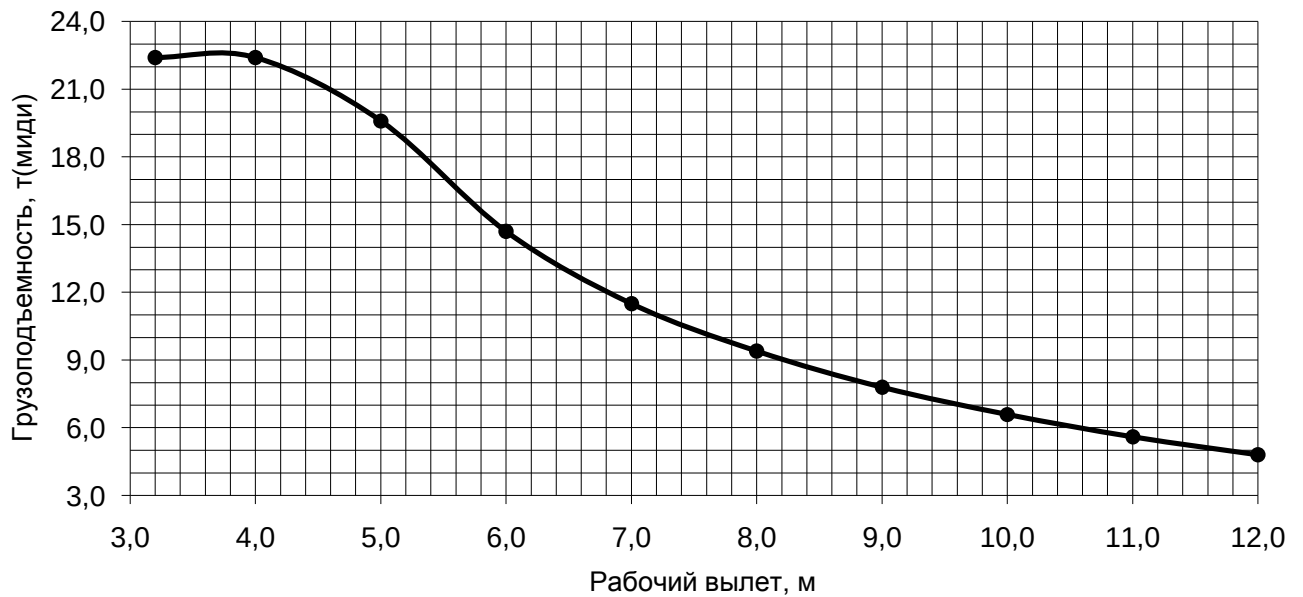
Грузовая характеристика. Лст=12,0-14,0м. \kappa=10 , противовес G=4,2 т.
