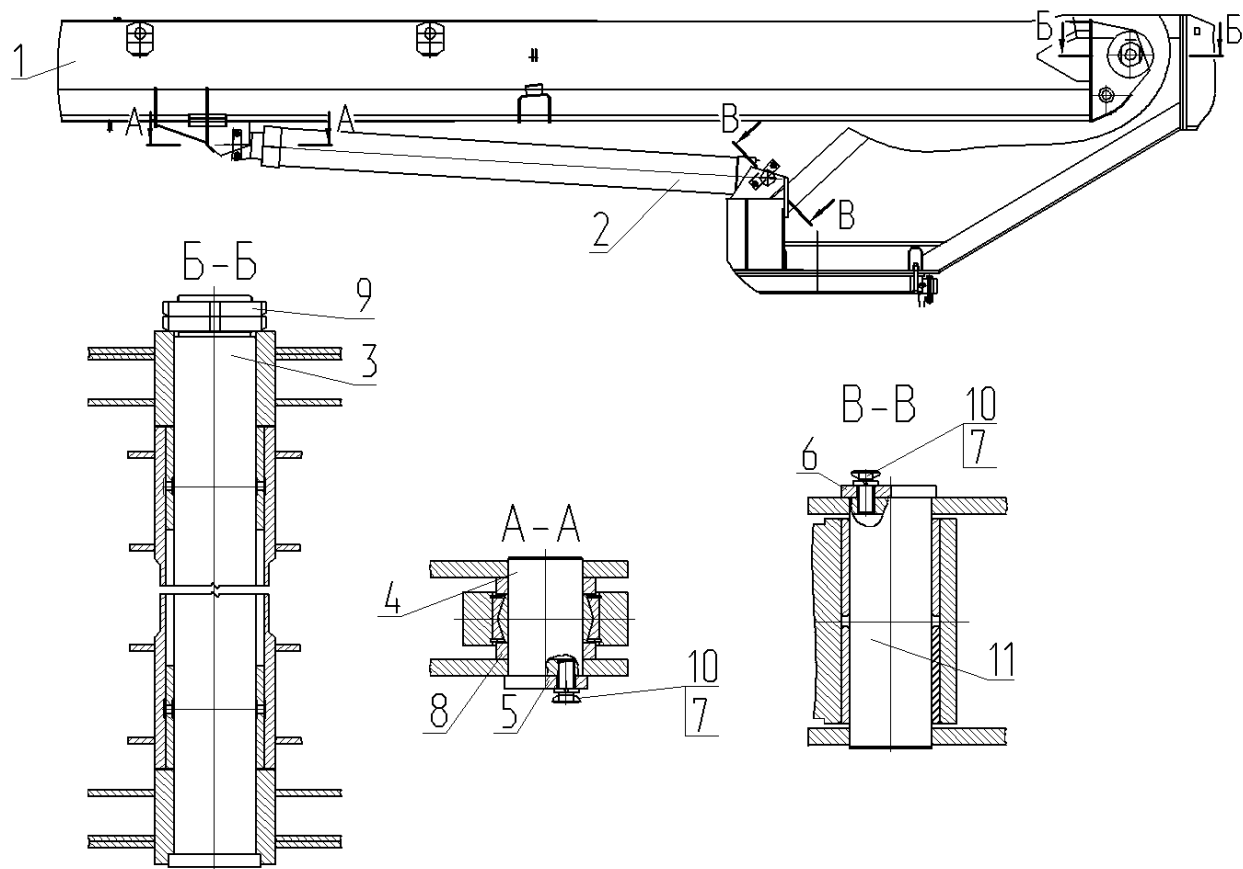
Рисунок 19 Рабочее оборудование
