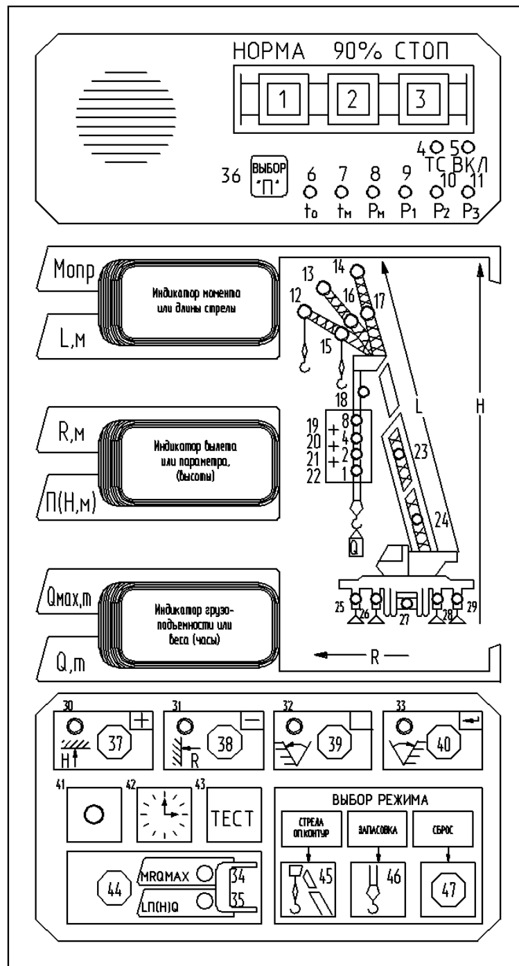
Рисунок 5 Лицевая панель ОНК
