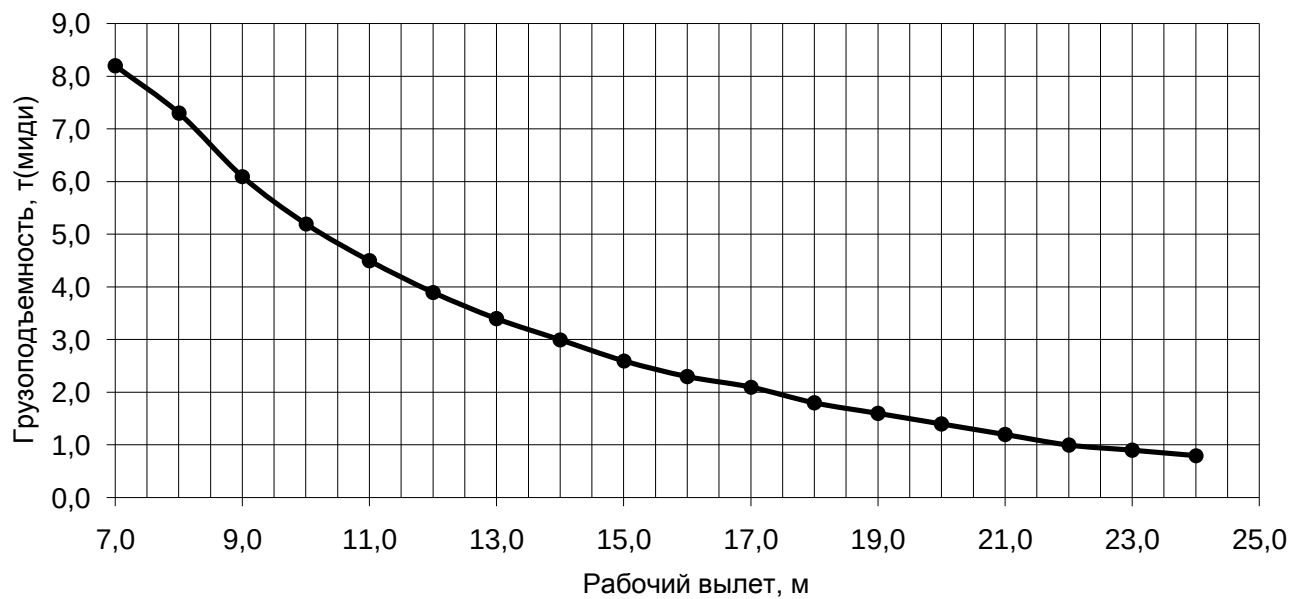
Грузовая характеристика. L_{ст}=26,0-28,0 м. \kappa=4 , противовес G=1,7 т.
