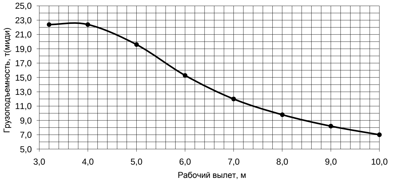
Грузовая характеристика. Лст=11,0-12,0м. \kappa=10 противовес G=4,2 т.
