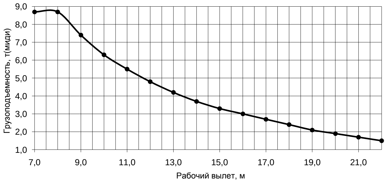
Грузовая характеристика. Лст=22,0-24,0м. \kappa=4 , противовес G=4,2 т.
