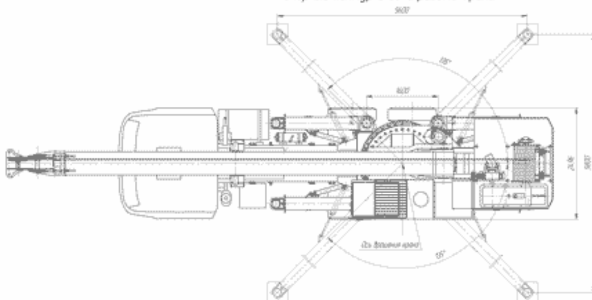
Опорный контур и зона работы крана
